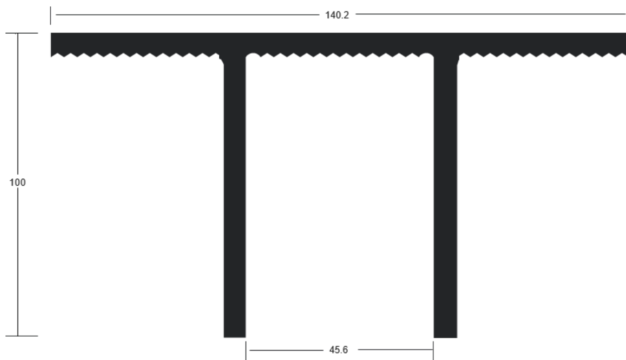
4507 Anclaje
