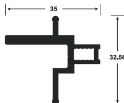
4504 Clip de sujeción horizontal
