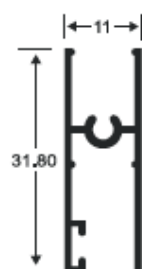
2624 HORIZONTAL MOVIL
