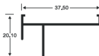
2626 RIEL SUPERIOR
