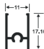
2625 HORIZONTAL FIJO
