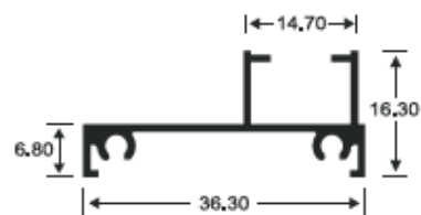
2629 MARCO FIJO
