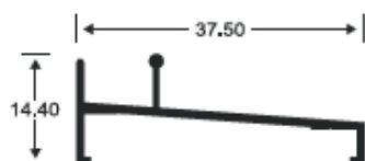
2627 RIEL INFERIOR
