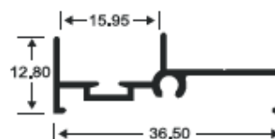
2628 MARCO MOVIL
