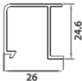
Junquillo Fijo (Monolítico 6-8mm) 7168
