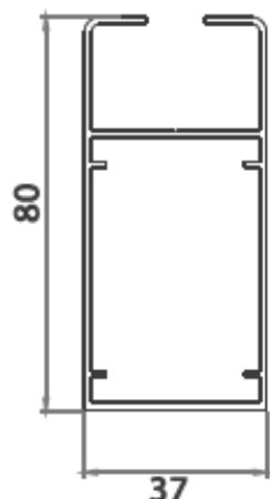
Montante Hoja Batiente (Monolítico) 7180
