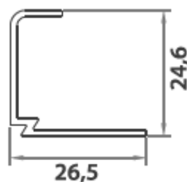
Junquillo Fijo (Insulado 24mm) 7169
