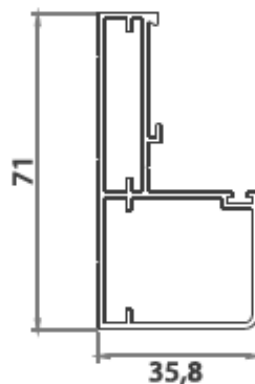
Marco Lateral Fijo 7111
