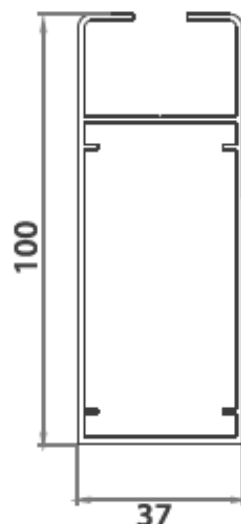
Montante Hoja Batiente (Monolítico) 7110
